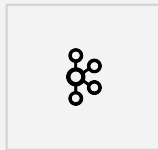
Apache Kafka
