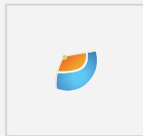
JSF
