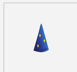
Dropwizard
