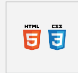
HTML/CSS
