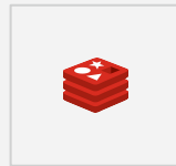
Redis
