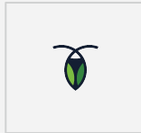
CockroachDB
